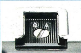
Zubehörschuh mit Mittenkontakt, umschaltbar auf X- und M-Blitzsynchronisation
